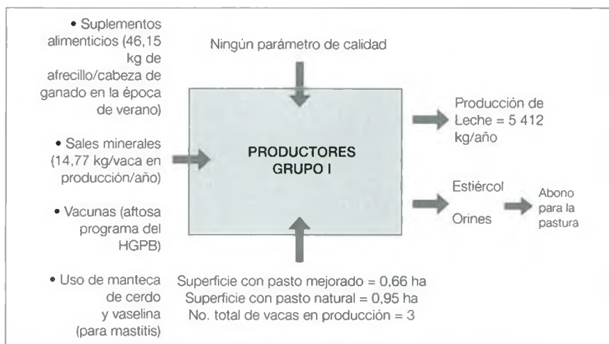
Figura 2. Caracterización de la función técnica de producción de leche del Grupo 1 en la microcuenca del río Illangama. Subcuenca del río Chimbo-Ecuador, 2009.
