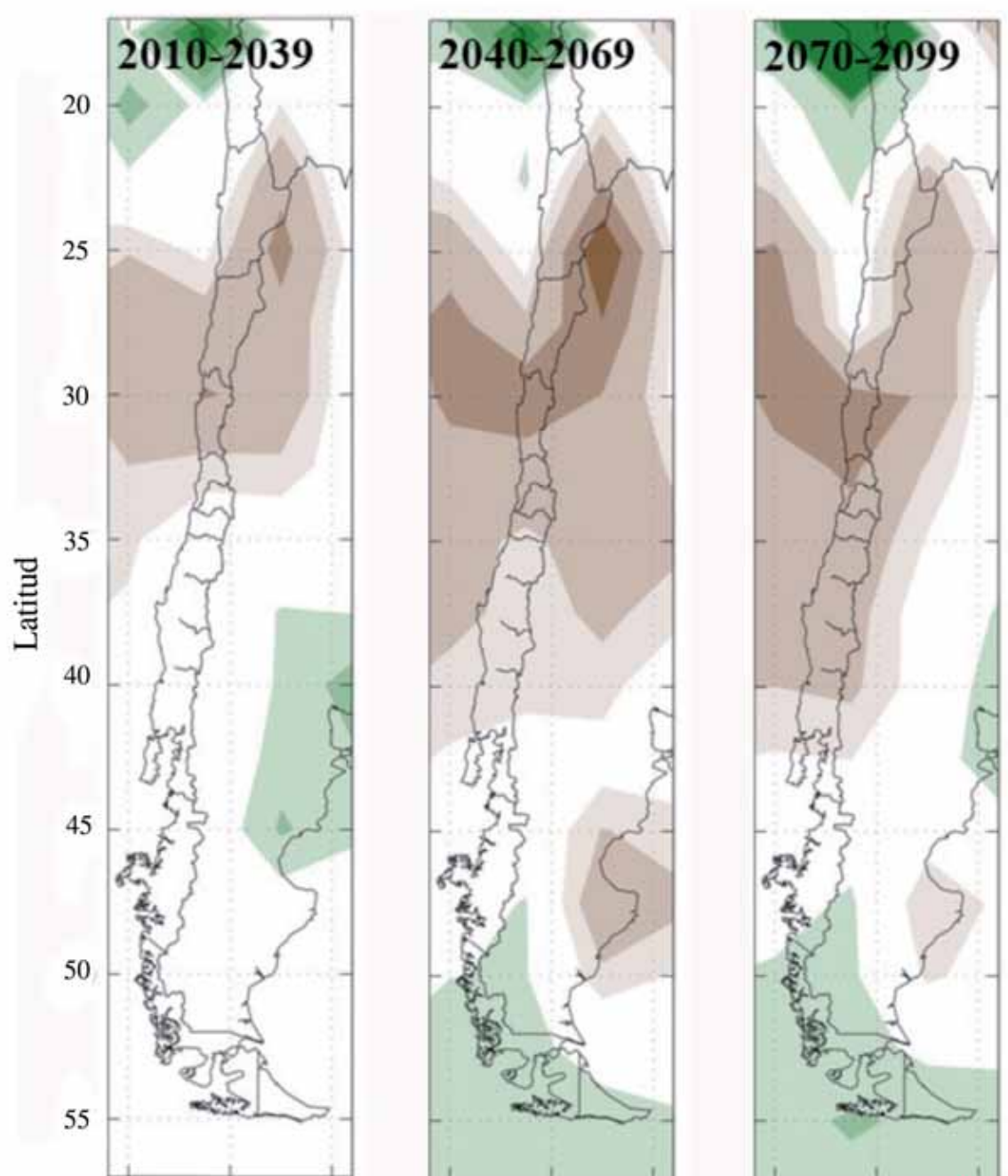
FIGURA 1.2 CHILE: PROYECCIONES DE TEMPERATURA PARA EL ESCENARIO B2 (Cambios en grados centígrados sobre base histórica)
