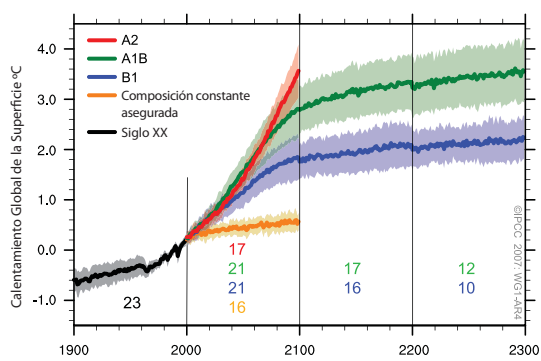
a) Cambio medio de la temperatura global
