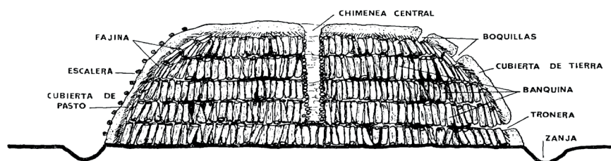
Figura 10 Corte vertical de un horno de carbón vegetal. (Dibujante: Aldo Barbieri.)
